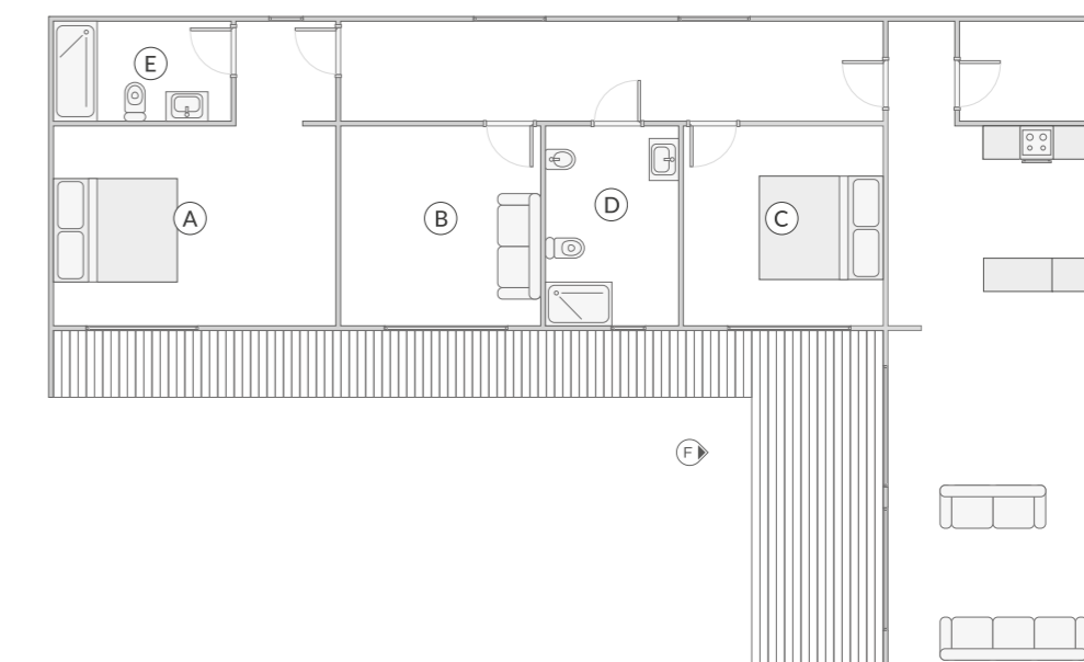
VISTA SUPERIOR VUE DE DESSUS ESCALA ÉCHELLE 1/150
